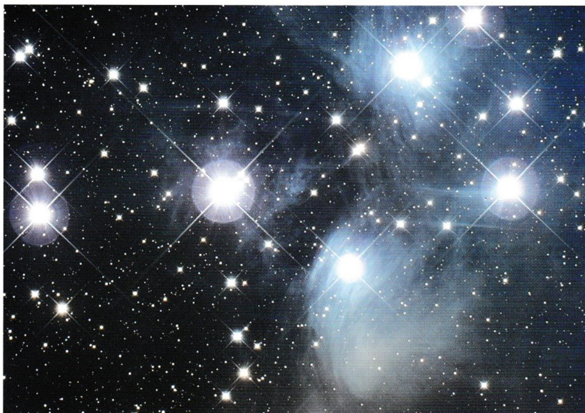
プレアデス星団
